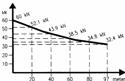
Tažná síla
